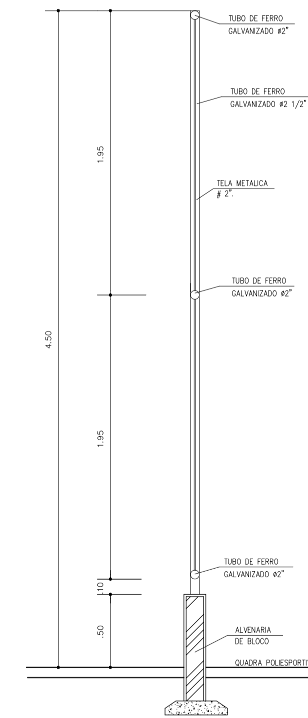
DET 11 ALAMBRADO / MURETA VISTA ESCALA 1/25
