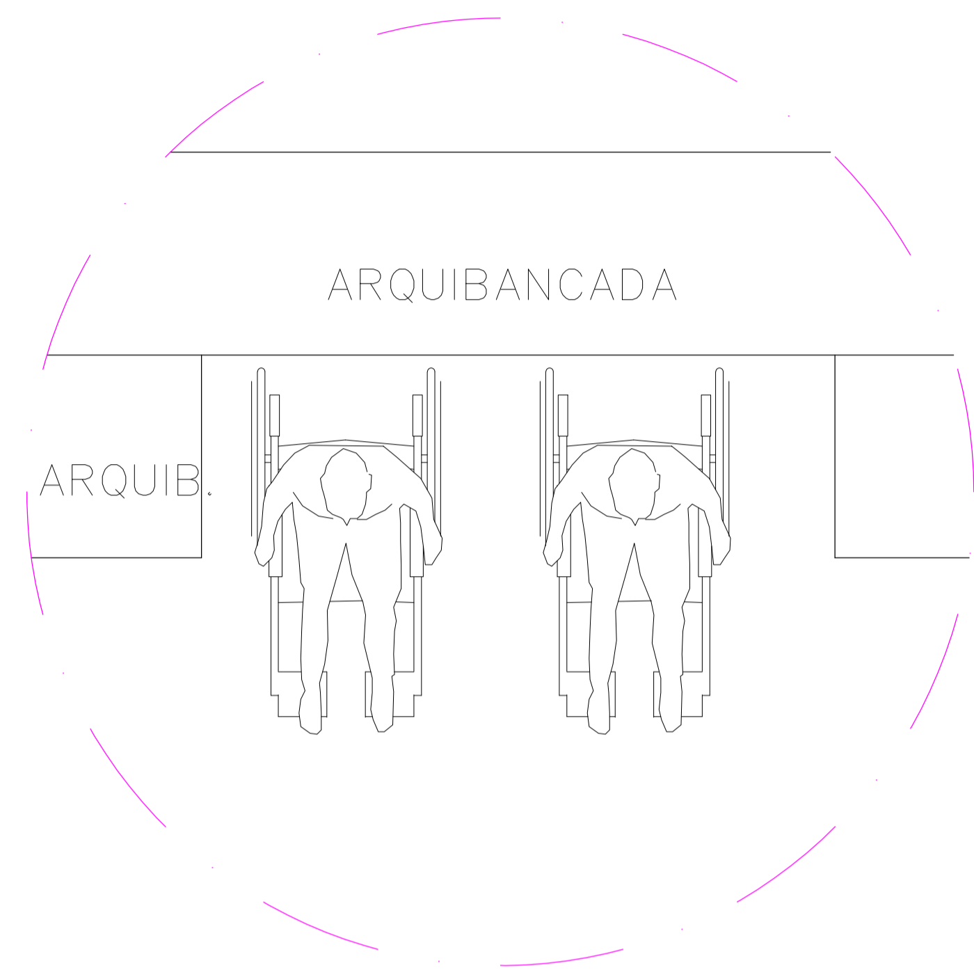
○ Detalle 2—espaço para Deficientes Esc. 1/10
